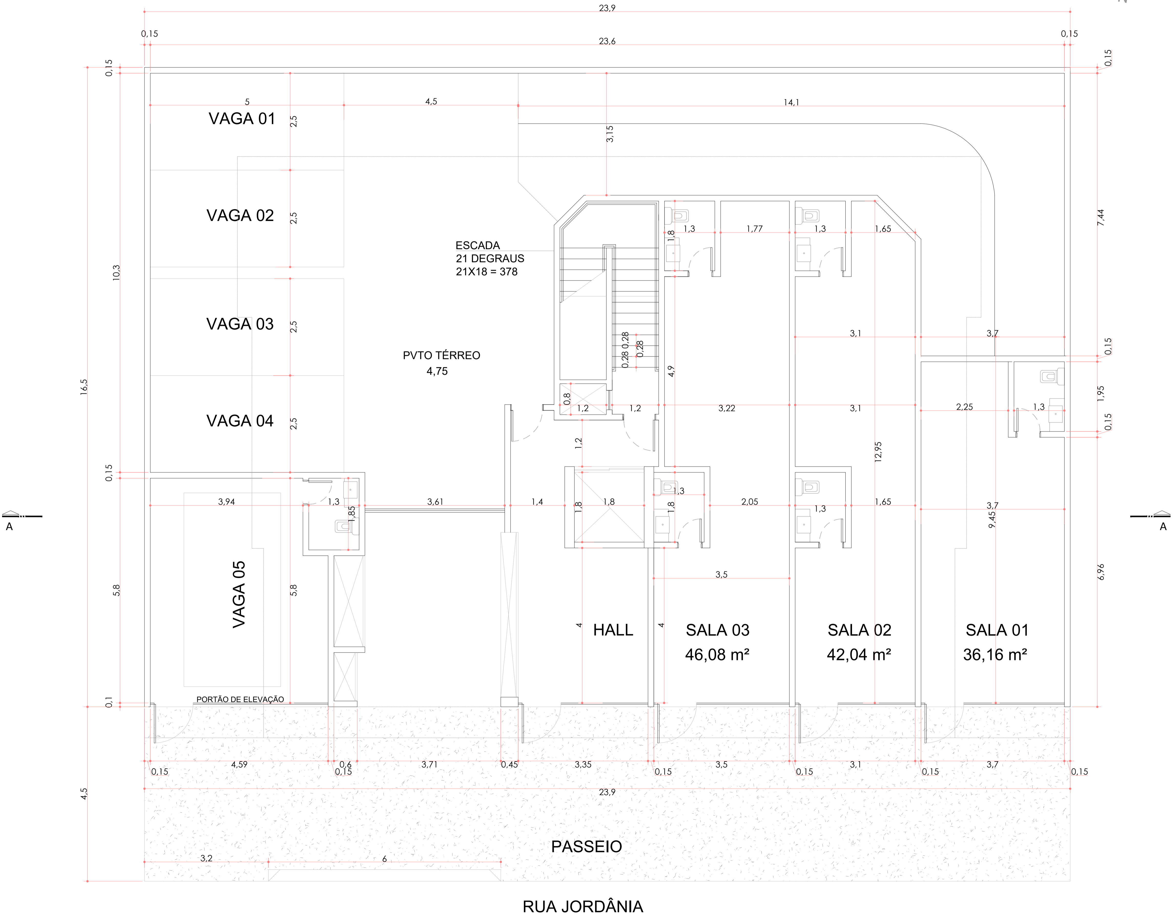
PLANTA BAIXA PAVIMENTO TÉRREO ESCALA 1:50
